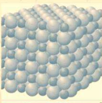
Ionic solid
